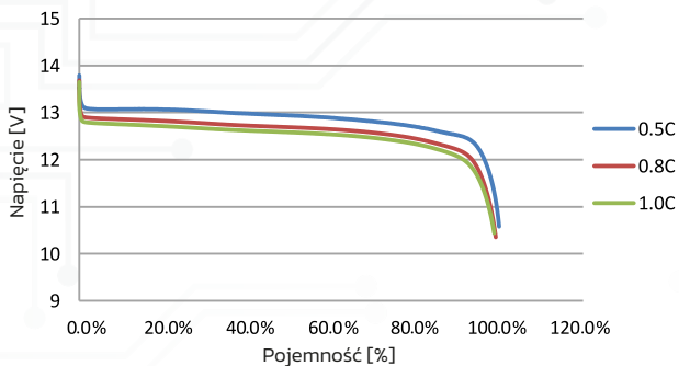
Krzywe rozładowania przy różnych zakresach @RT
