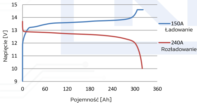
Charakterystyka ładowania 0,5C @RT
